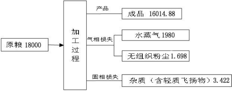
图2 本项目物料平衡图 单位 t/a
